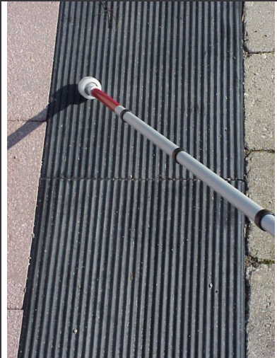
Abb. 13 f: Hartgummi-Rillenplatte (Hamburg) 0/3 mm Leitfunktion: 3,63 Aufmerksamkeitsf.: 3,32 (gute Ergebnisse mit Keramikspitzen, mangelhafte mit Rollspitzen) FüÙe: 6,00
