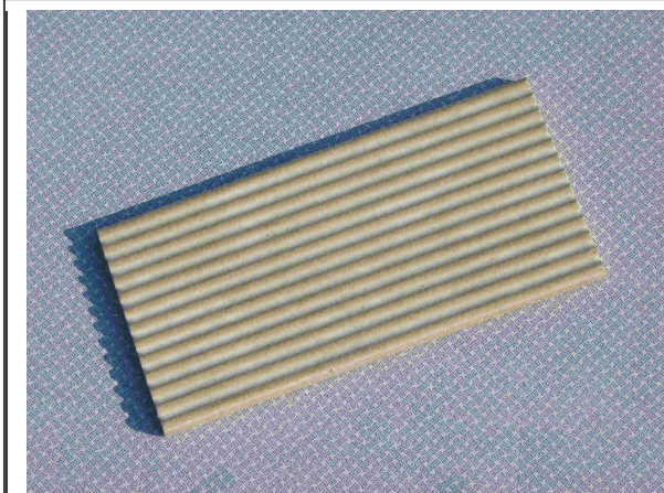
Abb. 4: Die Rillenstruktur mit einem Abstand von Rippe zu Rippe von ca. 10 mm belegte den zweitletztten Rangplatz. Sie erwies sich bei vielen Tests als so schlecht, dass sie ebenfalls als ungeeignet abzulehnen ist und aus der Norm gestrichen werden sollte.
