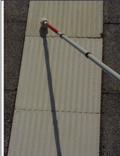
Abb. 13 d: Rillenstruktur (Berlin) 20/4 mm Leitfunktion: 3,34 Aufmerksamkeitsf.: 4,33 FüÙe: 6,00
