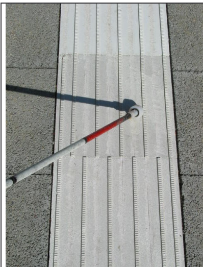
Abb. 11d: Hobis (Ebersbach) 60/3,5 mm Leitfunktion: 1,82 Füße: 2,50
