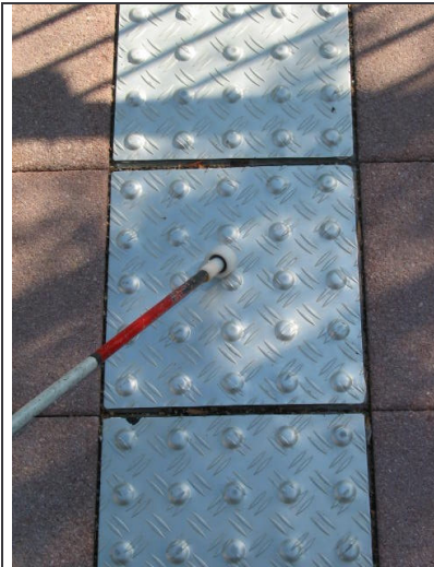
Abb. 11a: Klangtegels (Noppenblech, Holland); 57/4,5 mm Aufmerksamkeitsf.: 1,10
