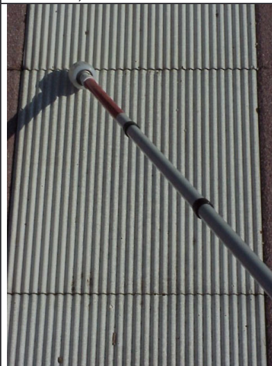
Abb. 13 h: Rillenstruktur (Hamburg) 10/3 mm Leitfunktion: 3,90 Aufmerksamkeitsf.: 4,95 FüÙe: 6,00
