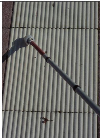
Abb. 13 g: Rillenstruktur (Berlin) 15/4 mm Leitfunktion: 3,65 Aufmerksamkeitsf.: 4,47 FüÙe: 6,00
