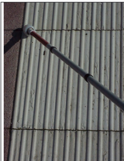
Abb. 13 a: Rippenstruktur 20/2,5 mm Leitfunktion: 2,94 Aufmerksamkeitsf.: 3,69 FüÙe: 5,83
