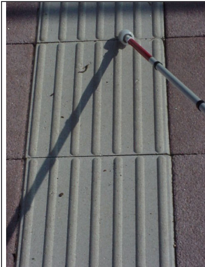
Abb. 12 a: Geleidelijn ("halbe Zigarren"; Niederlande) 45/5 mm Leitfunktion: 2,41 Aufmerksamkeitsf.: 2,65 Füße: 3,36
