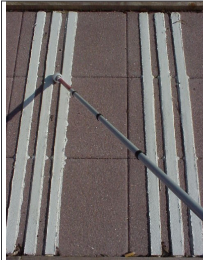
Abb. 12 g: Kaltplastik: Adidas-Streifen (Schweiz) 60/6,5 mm Leitfunktion: 2,76 Aufmerksamkeitsf.: 2,56 FüÙe: 3,74
